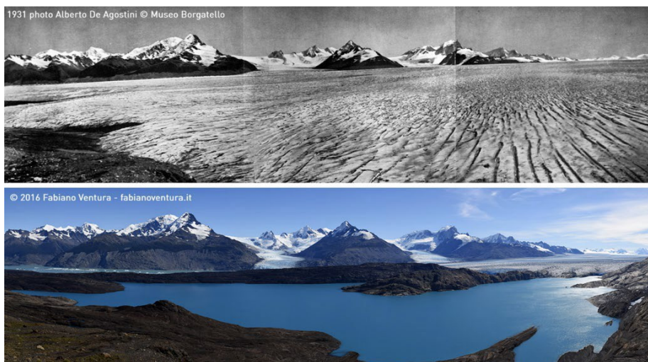
Fig. 2. Comparación de fotografías del Glaciari Upsala, en Argentina tomadas en los años 1931 y 2016.
