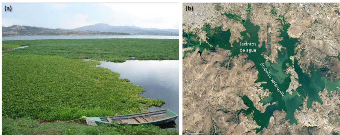
Fig. 1. Foto de jacintos de agua en el Embalse Valsequillo, México (a). Imagen del satélite Landsat 8 tomada el 9 de enero de 2020 (b) que muestra la superficie del mismo embalse cubierta por jacintos de agua.
