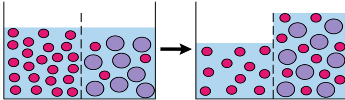
Figura 2 Ósmosis. Los puntos rojos representan agua y el punto violeta son las partículas de soluto. Las moléculas de agua atraviesan la membrana para reducir la concentración de la solución. Observe cómo las partículas de soluto no pueden atravesar la membrana. Fuente: https://www.science-sparks.com/wp-content/uploads/2018/09/Osmosis-Diagram-1536x536.jpeg
