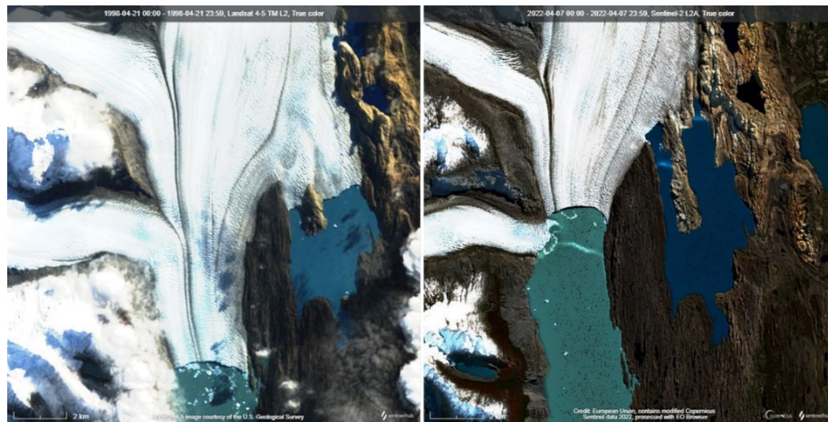
Fig. 3. Imágenes satelitales del Glaciar Upsala , en Argentina. La imagen reciente Sentinel-2 L2A de abril 2022 (derecha) muestra la pérdida de hielo en el frente del glaciar y en los bordes al compararla con la imagen Landsat 4-5 TM L2 de abril 1998 (izquierda)
