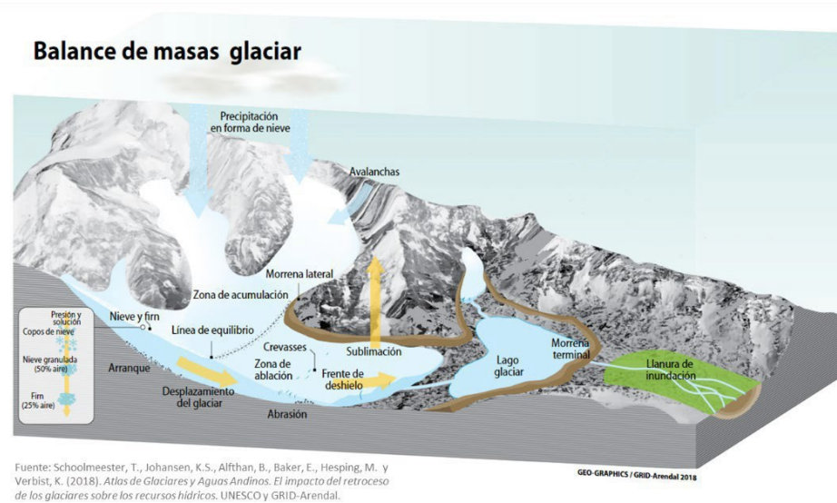
Fig. 1. Zonas de acumulación y ablación de nieve en un glaciari.
