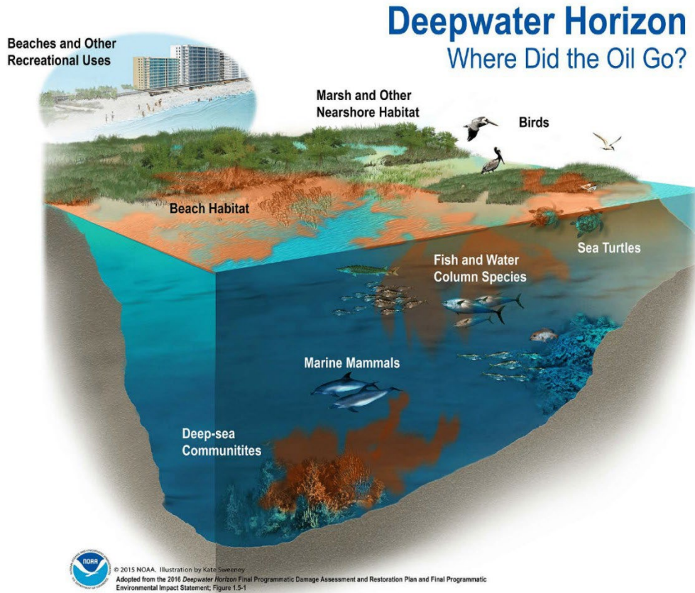
Figura 3 Derrame de petróleo de Deepwater Horizon. Fuente: NOAA 2015
