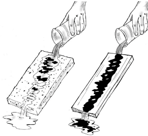
Figura 2 Agua que atraviesa un "humedal saludable" frente a un "humedal dañado".
